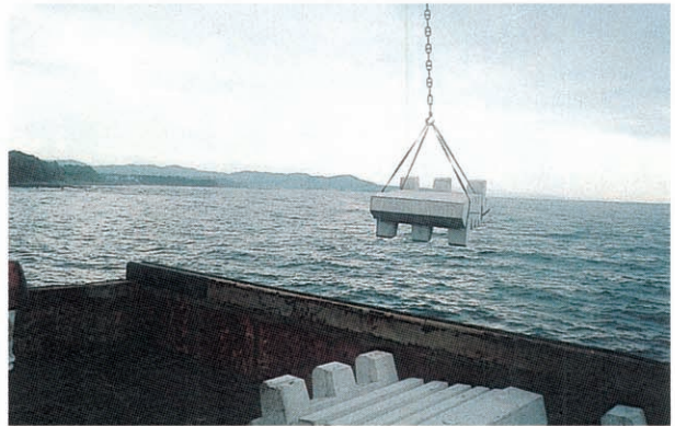
魚礁の設置
